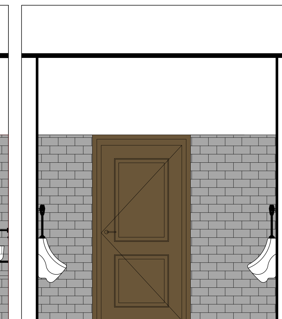
ŚCIANA 8-8
