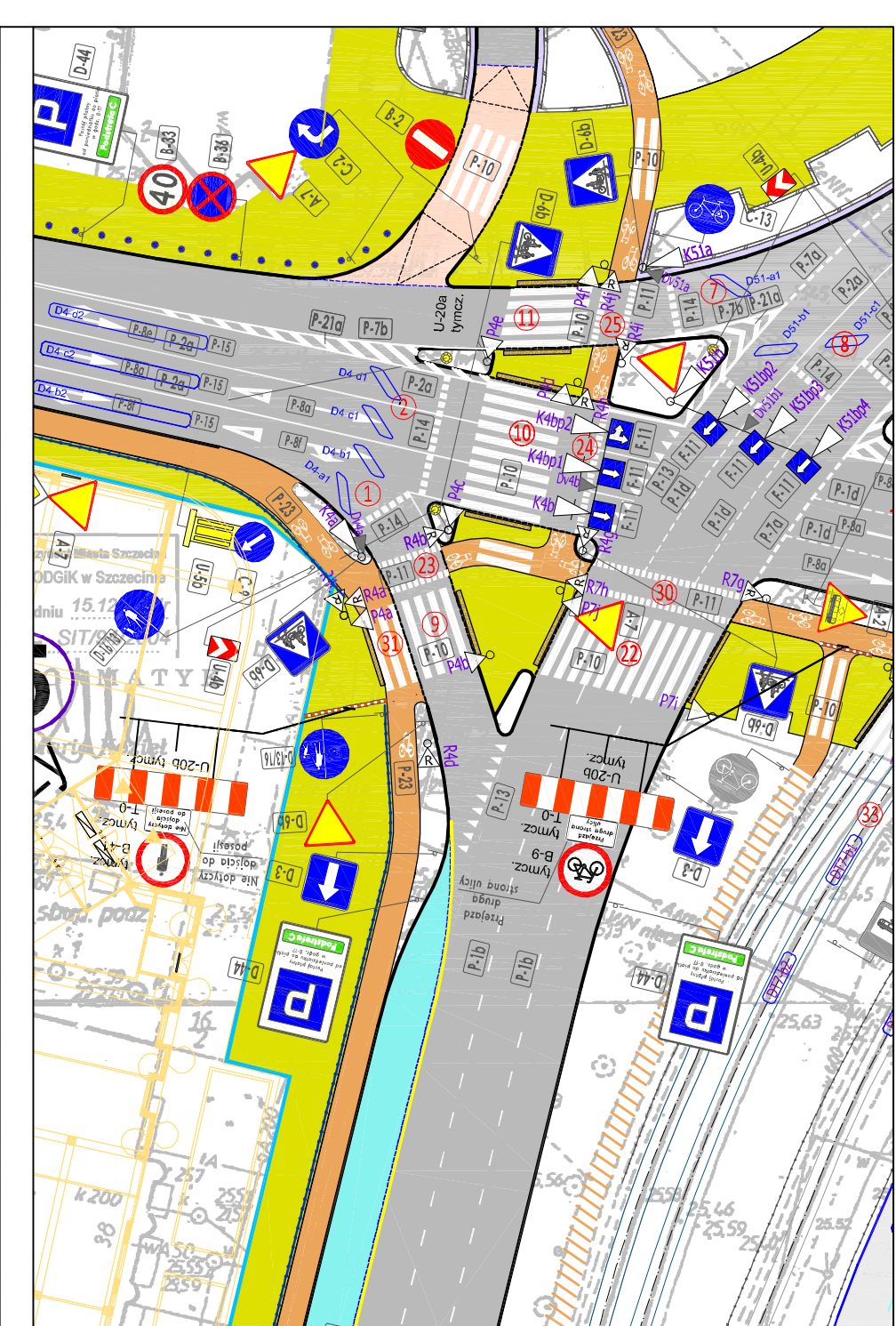
Zamknięcie istniejącej ścieżki rowerowej i chodnika na Placu Żołnierza - skala 1:500
