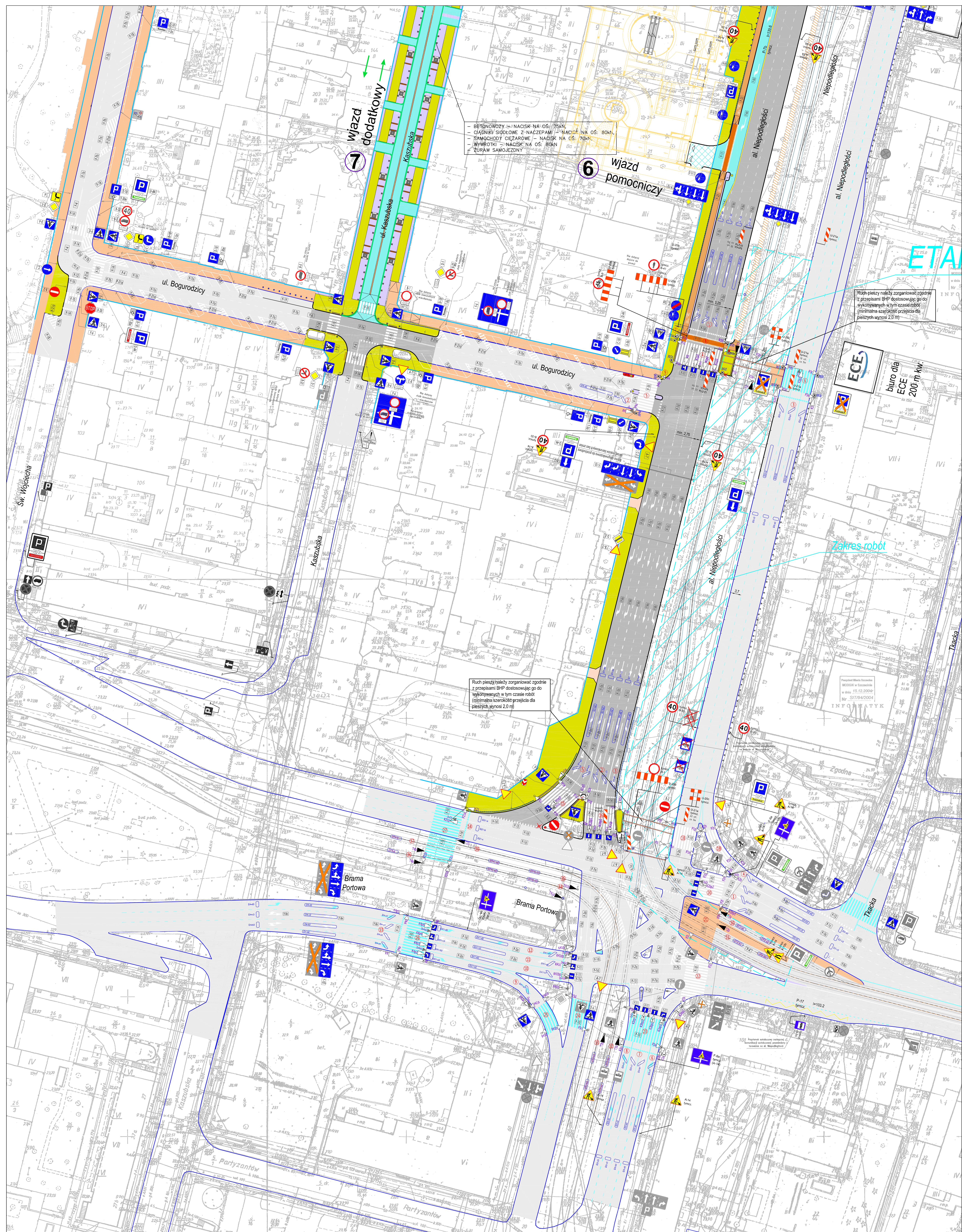
Zamknięcie istniejącej ścieżki rowerowej i chodnika na Placu Żołnierza - skala 1:500
