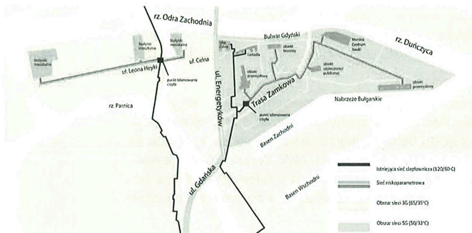
Rysunek nr 1. Schemat sieci niskoparametrowej na terenach Łasztowni oraz Kępy Parnickiej
