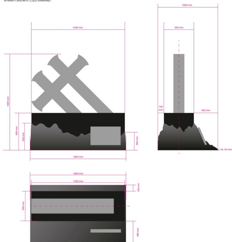
WYMIARY CAŁKOWITE I CZĘŚCI KAMIENNEJ
