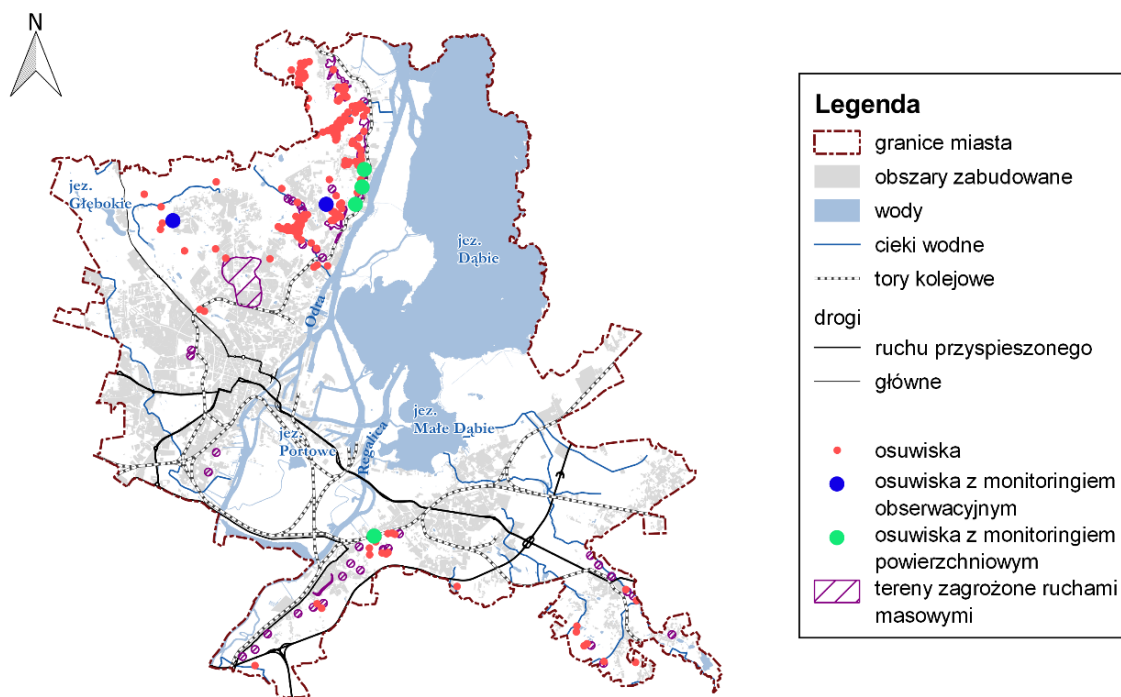
Rysunek 11 Mapa osuwisk i terenów zagrożonych ruchami masowymi na terenie miasta Szczecin 69
