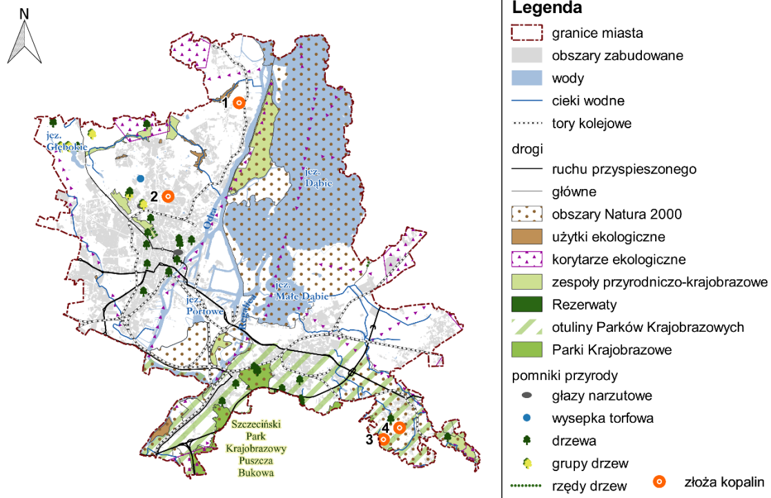
Rysunek 13 Mapa z lokalizacją złóż kopalin oraz obszarów chronionych w granicach miasta Szczecin
